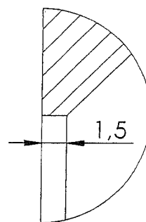
Детайл А Мащаб 10 : 1
