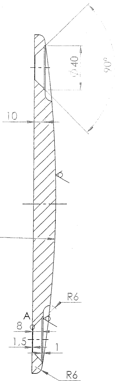
A-A 1 : 2
