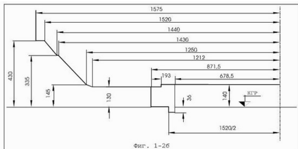
Фиг. 1-26. Статичен габарит на подвижния железопътен състав 0-ВМ (03-Т) долна част - за железопътни линии с междурелсие 1520 mm. Вертикалните размери се отнасят за обресорените части. За необресорените части тези размери се намаляват с 15 mm. Долната част на статичния габарит на подвижния железопътен състав за международни съобщения (03-Т) съответства на габарит 03-ВМ.
