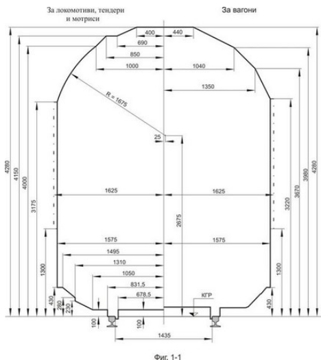
Фиг. 1-1. Статичен габарит на подвижния железопътен състав за международни съобщения 03-ВМ (03-Т) - горна част.
