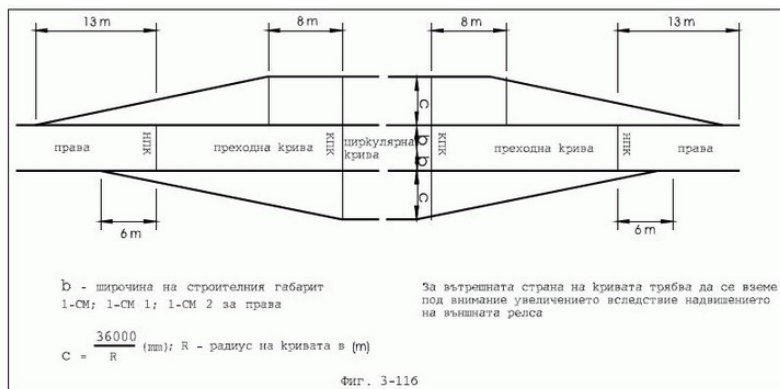
Фиг. 3-11б. Преход на строителните габарити 1-СМ, 1-СМ 1 и 1-СМ 2 от права в преходна и циркулярна крива (при циркулярна крива с преходни криви)
