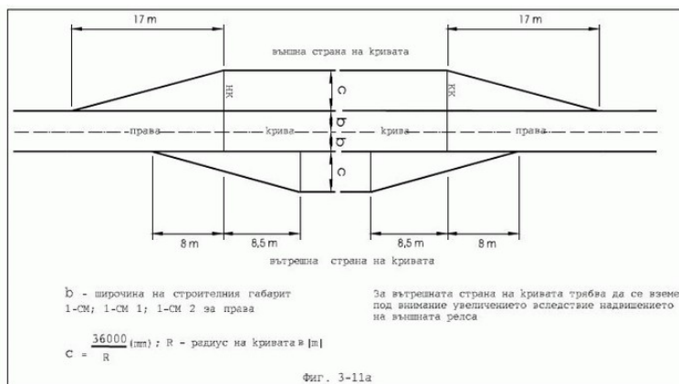
Фиг. 3-11а. Преход на строителните габарити 1-СМ, 1-СМ 1 и 1-СМ 2 от права в преходна и циркулярна крива (при циркулярна крива без преходни криви)
