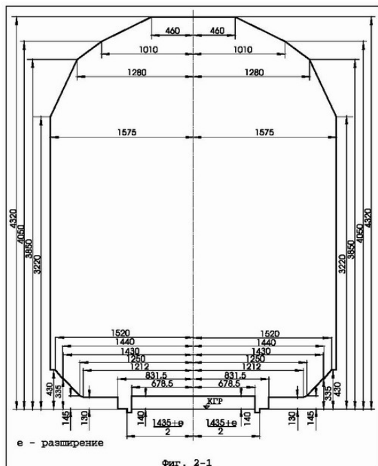
Фиг. 2-1. Статичен габарит на натоварването "А"
