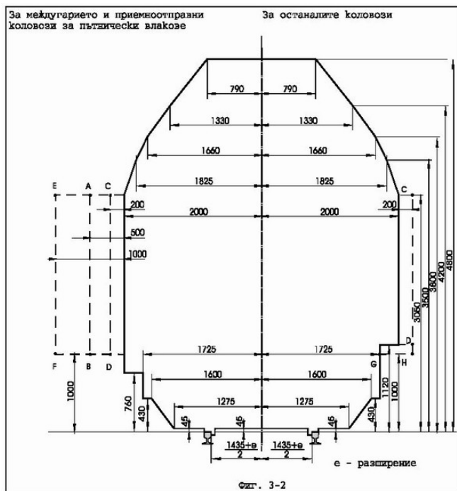
Фиг. 3-2. Строителен габарит 0-СМ за прави и криви с R ? 250 m. В участъците, където е обозначен "Строителен габарит 0-СМ за прави и криви с R ? 250 m", може да се движи подвижен състав, отговарящ на: - статичен габарит на подвижния състав за международни съобщения 03-ВМ (03-Т) - фиг. 1-1 от приложение № 1; - статичен габарит на подвижния състав за вътрешни съобщения 02-ВМ (02-Т) - фиг. 1-3 от приложение № 1; - статичен габарит на подвижния състав за 0-ВМ (01-Т) - фиг. 1-4 от приложение № 1; - габарит на натоварването "А" - фиг. 2-1 от приложение № 2.
