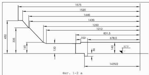
Фиг. 1-2а. Статичен габарит на подвижния железопътен състав 0-ВМ (03-Т) долна част - за железопътни линии със стандартно междурелсие 1435 mm. Вертикалните размери се отнасят за обресорените части. За необресорените части тези размери се намаляват с 15 mm. Долната част на статичния габарит на подвижния железопътен състав за международни съобщения (03-Т) съответства на габарит 03-ВМ.
