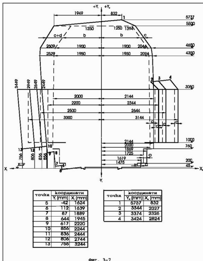
Фиг. 3-7. Строителен габарит 1 - СМ 2 за жп линии в крива с надвишение на външната релса (при ново строителство и преустройства) - - - - - Очертание на строителния габарит 1-СМ2 за коловоз в права --- Основно очертание на строителния габарит 1-СМ 2 за коловоз в крива
