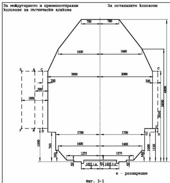
Фиг. 3-1. Строителен габарит на съществуващите жп линии за прави и криви с R ? 250 m. В участъците, където е обозначен "Строителен габарит на съществуващите жп линии за прави и криви с R ? 250 m", може да се движи подвижен състав, отговарящ на:
