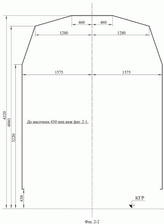
Фиг. 2-2. Статичен габарит на натоварването "В"
