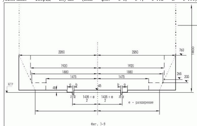
Фиг. 3-9. Строителен габарит 1-СМ 2 за стоманени жп мостове система
