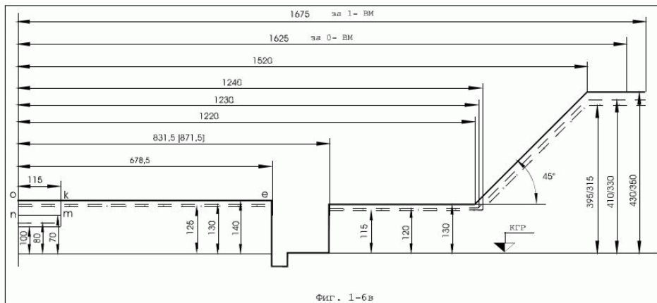
Фиг. 1-6в. За возила, които могат да преминават през механизирани гърбици, със спирачки стар тип. - - - За обресорените части на коша. - - - За части, закрепени на обресорената рама на талигата. -х-х-х- За необресорени части. Размерите, посочени с дроб, означават: - в числителя - размери, които трябва да притежават всички новостроящи се, предназначени за международно съобщение вагони, също така и по-рано построени вагони при движение по железопътните линии на Република България, Република Унгария, Република Полша, Румъния, Чешката Република и Република Словакия; - в знаменателя - размерите на по-рано построени вагони при движението им в границите на железопътните линии с междурелсие 1520 mm. Размерите, посочени в скоби, вадат за железопътни линии и коловози с междурелсие 1520 mm. Вагоните на всички членове на Спогодбата за международно железопътно пътническо съобщение (СМПС) и СМГС, които имат очертание по линията о-к-е (фиг. 1-6в), могат да преминават през гърбици при произволно положение на механизирания спирачка (вагонозадържател), вкл. работно положение. Вагони, имащи долно очертание о-п-ш-к-е (фиг. 1-6в), могат да се пропускат през механизирани спирачки - стар тип, само при неработно положение на последните. Механизираният спирачки стар тип трябва във всички случаи, когато това е възможно, да се преустрой в съответствие със строителен габарит 1-СМ2 (приложение 3, фиг. 3-10), така че да могат да преминават вагони с долно очертание по фиг. 1-6в.
