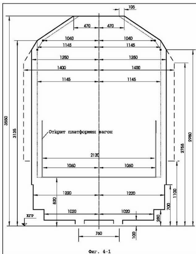
Фиг. 4-1. Статичен габарит на подвижния железопътен състав при 760 mm жп линии --- Очертание на габарита на возилата ..... Ограничителна линия на товарите - - - - - Габарит на странично поставените сигнални фенери.
