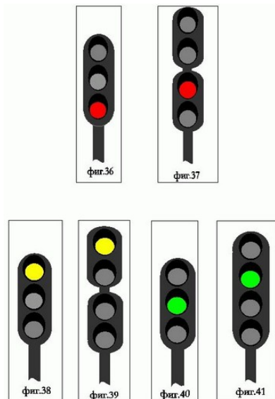
Изходни светофори по скоростната сигнализация
