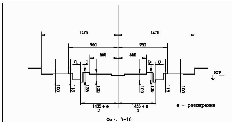
Фиг. 3-10. Строителен габарит 1-СМ 2 (долна част) за вагонозадържатели в права* (при ново строителство и преустройства)
