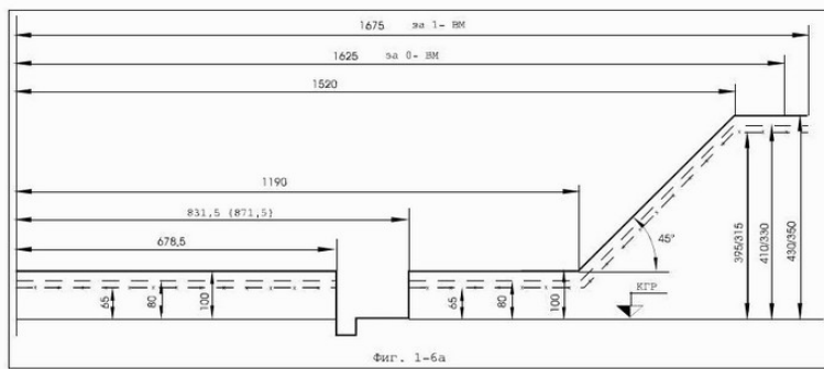
Фиг. 1-6а. Статичен габарит на подвижния железопътен състав 0-ВМ (01-Т) и 1-ВМ (0-Т) - долна част. За возила, които не могат да преминават през механизирани гърбици.
