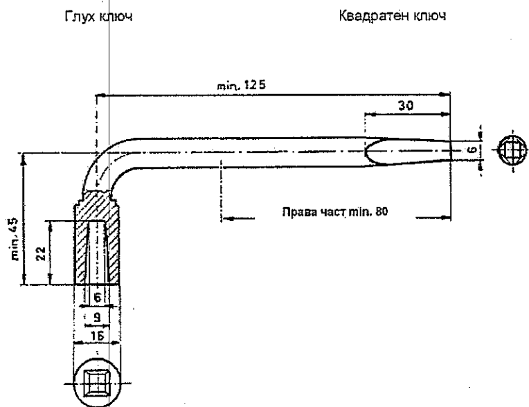
Фиг. 1 Ключ квадрат
